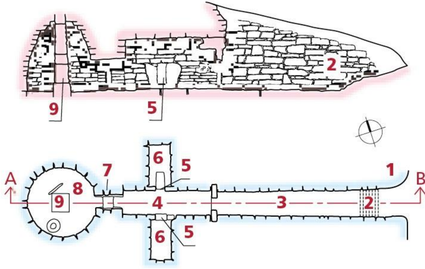
Sezione AB
